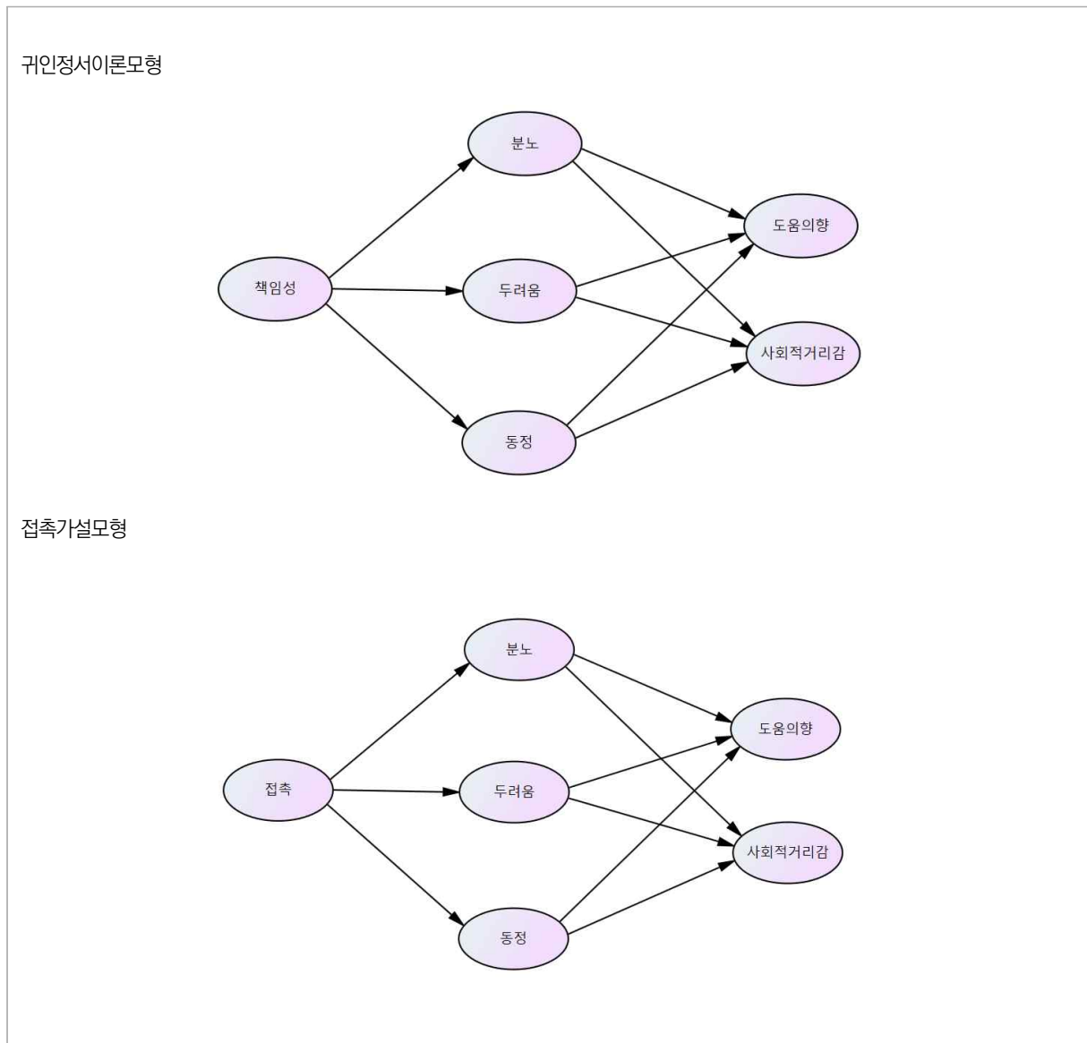
그림 1. 연구 모형
